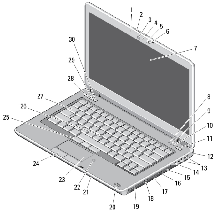
그림 1. 전면 모양
